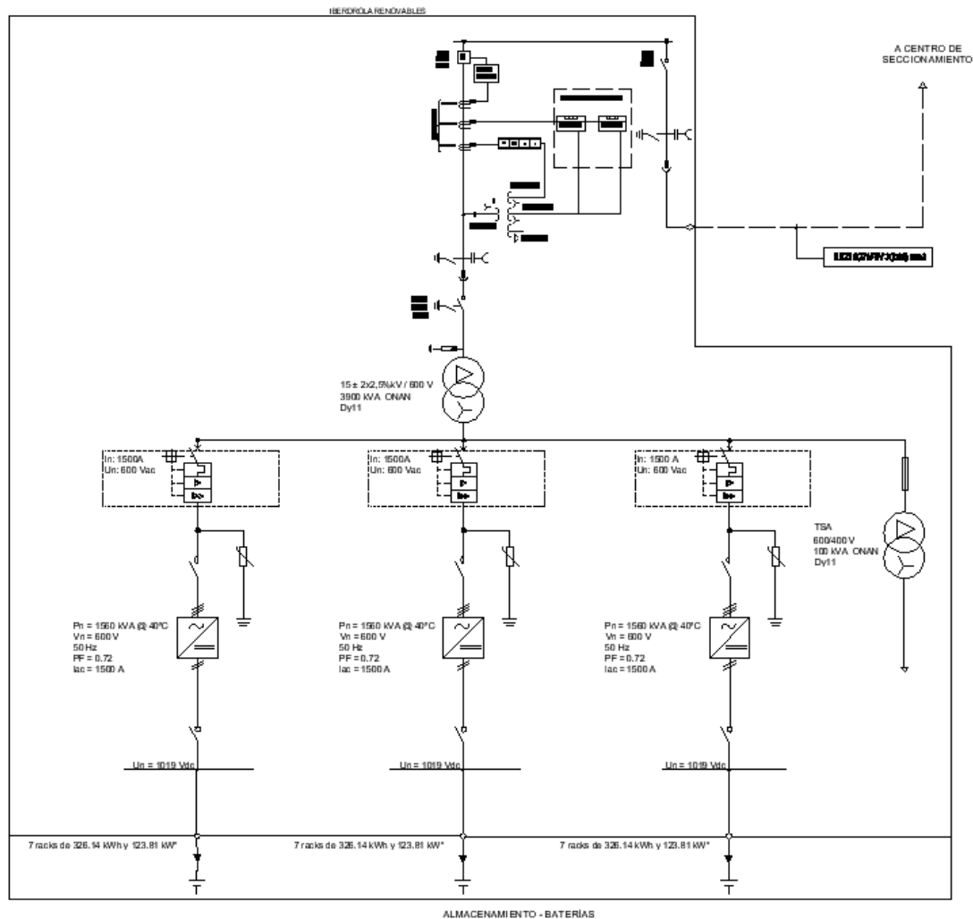
Imagen del unifilar general
