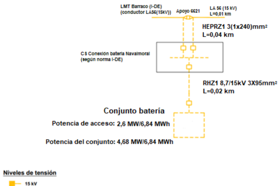
Imagen de esquema eléctrico simplificado mm 2
